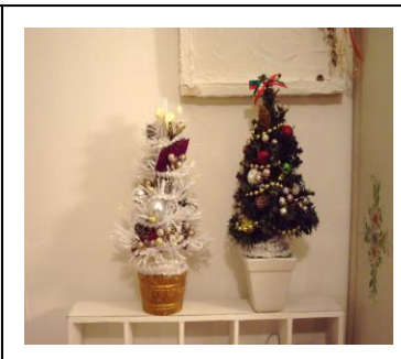
ツリー例
